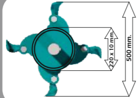
DIAMETRO EJE Ø 60 mm. AXLE DIAMETER Ø 60 mm. DIAMÈTRE DE L'AXE Ø 60 mm. ACHSDURCHMESSER Ø 60 mm.
