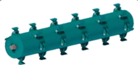
ROTOR MARTILLO OSCILANTE, BAJA ABSORCIÓN DE POTENCIA SWINGING HAMMER ROTOR, LOW POWER ABSORPTION ROTOR MARTEAUX OSCILLANTS, FAIBLE ABSORPTION DE PUISSANCE ROTOR MIT BEWEGLICHEN HÄMMERN, NIEDRIGE LEISTUNGS-AUFNAHME
