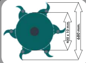
DIAMETRO EJE Ø 75 mm. AXLE DIAMETER Ø 75 mm. DIAMÈTRE DE L'AXE Ø 75 mm. ACHSDURCHMESSER Ø 75 mm.
